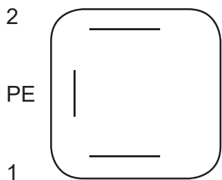
E-konektor PG09 - DIN43650
